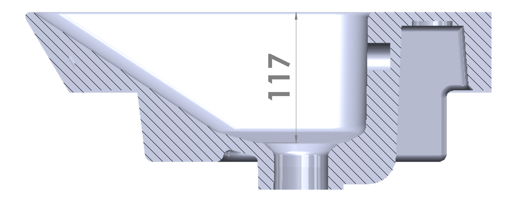
SEZIONE A-A SCALA 1:2
